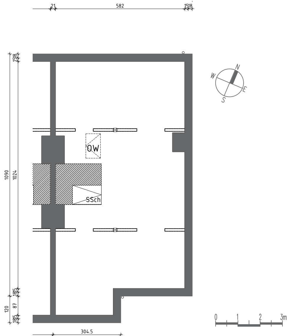
PODDASZE NIEUŻYTKOWE skala 1:100 pow. podłogi – 59,80m 2
